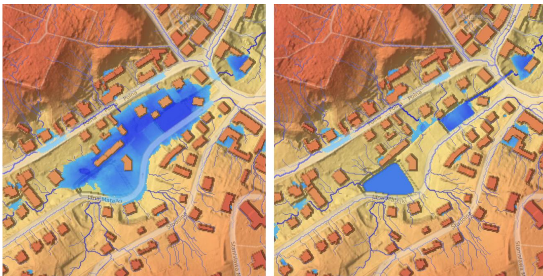
Ryc. 6.4.1.10. Sytuacja podtopień terenu przed (lewy rysunek) i po przeprowadzeniu prac hydrotechnicznych przy opadzie 20 mm przez 30 min.
