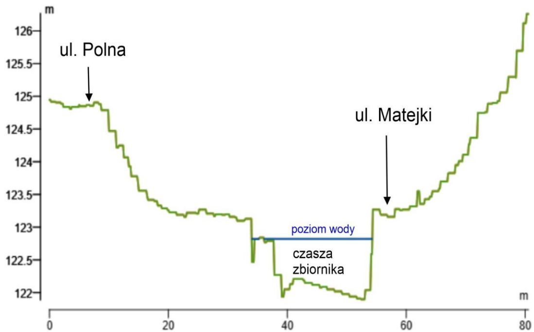
Ryc. 6.4.1.3. Profil poprzeczny przez zbiornik i jego otoczenie w warunkach braku opadów - stan istniejący.
