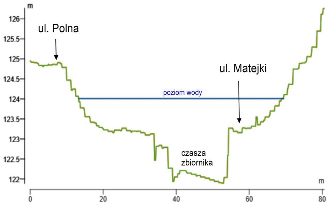
Ryc. 6.4.1.4. Profil poprzeczny przez zbiornik i jego otoczenie w warunkach opadów 20 mm przez 30 min - stan istniejący. Poziom wody wzrasta o przeszło 120 cm i podtapia ul. Matejki.
