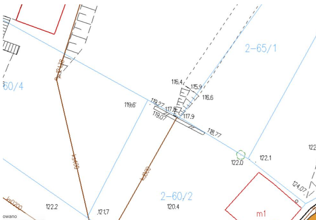
Ryc. 6.4.1.7. Fragment mapy zasadniczej z uzbrojeniem terenu dla odcinka wylotu wód z rurociągu 800 mm do rowu otwartego.
