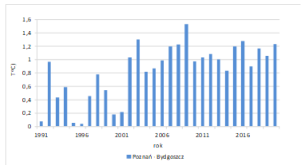
Rys. 2.2.2. Przebieg temperatury w Poznaniu i Bydgoszczy w wieloleciu 1991-2020: a) – w przebiegu rocznym, b) – różnice średniej rocznej temperatury, c) w okresie wegetacyjnym, d) – różnice średniej temperatury w okresie wegetacyjnym. Źródło: ITP Oddział Bydgoszcz na podstawie danych IMGW-PIB.
