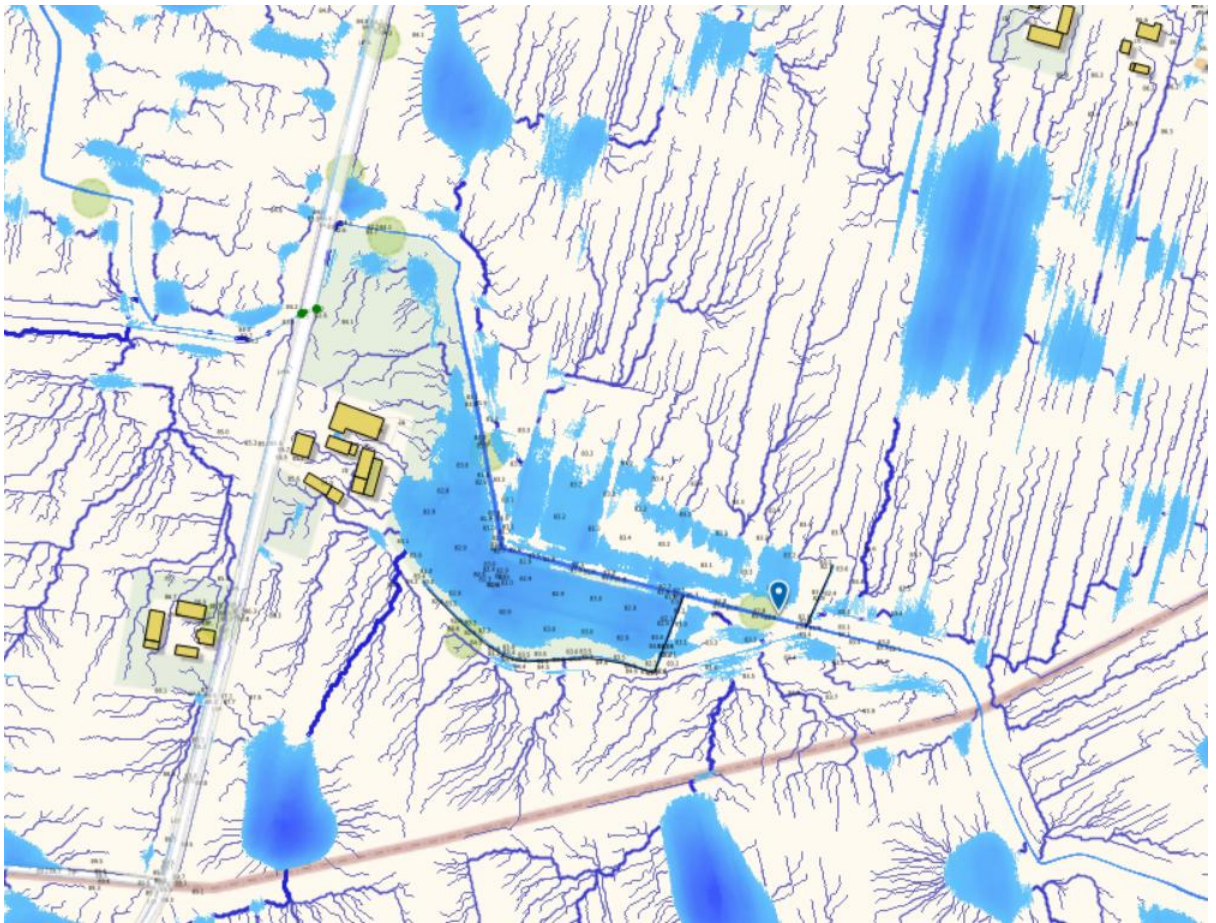
Ryc. 6.4.1.2. Lokalizacja analizowanego rowu na tle mapy głównych ścieżek spływu wód opadowych i roztopowych podczas opadów 10 mm
