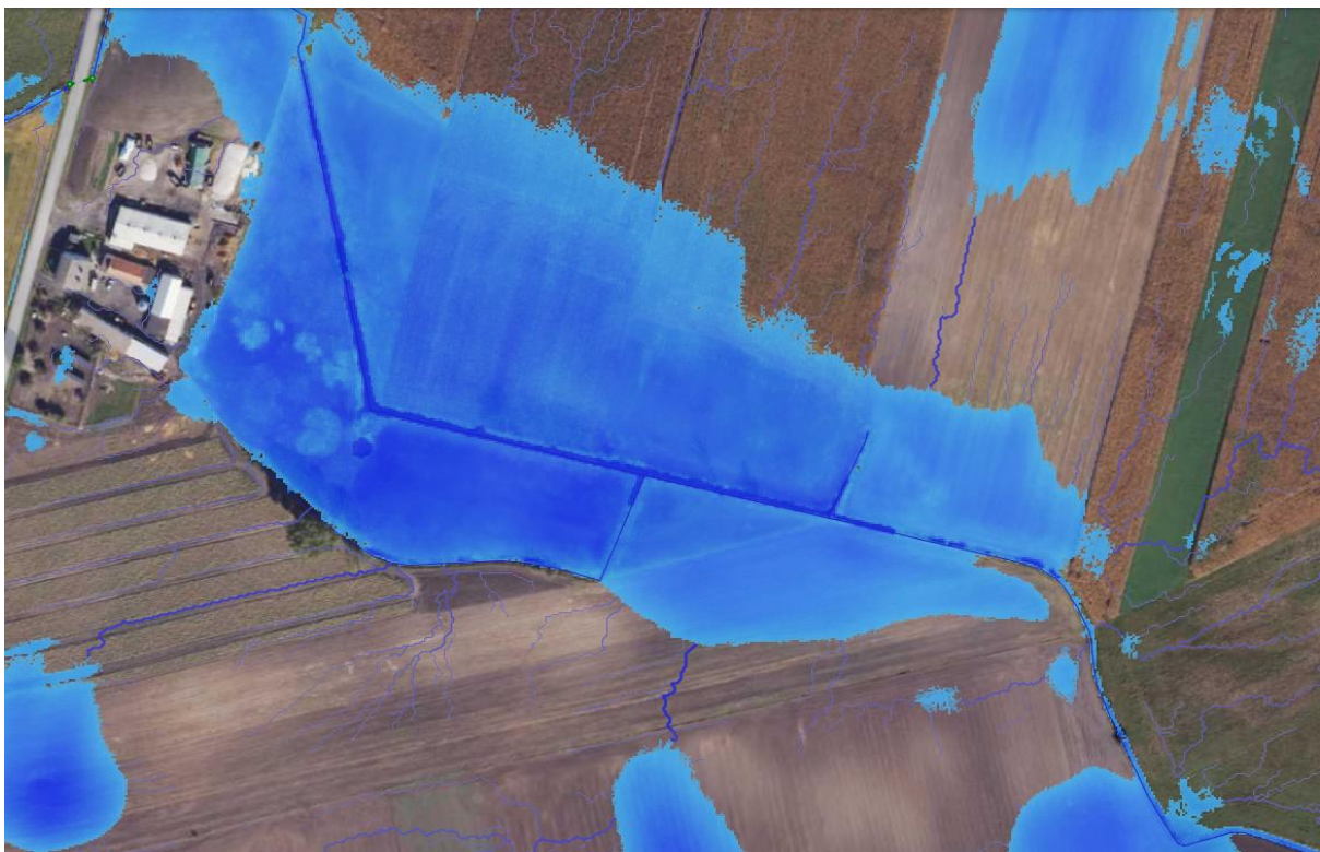
Ryc. 6.4.1.4. Zasięg zalewu wód w otoczeniu analizowanego cieku (bez zbiorników) podczas opadów 20 mm
