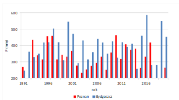
Rys. 2.2.1. Przebieg opadów w Poznaniu i Bydgoszczy: a) – roczne sumy opadów atmosferycznych, b) – różnice rocznych sum w wieloleciu 1991-2020, c) sumy opadów atmosferycznych w okresie wegetacyjnym, d) – różnice sum opadów atmosferycznych w okresie wegetacyjnym. Źródło: ITP Oddział Bydgoszcz na podstawie danych IMGW-PIB.
