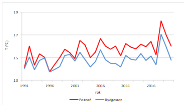
Rys. 2.2.2. Przebieg temperatury w Poznaniu i Bydgoszczy w wieloleciu 1991-2020: a) – w przebiegu rocznym, b) – różnice średniej rocznej temperatury, c) w okresie wegetacyjnym, d) – różnice średniej temperatury w okresie wegetacyjnym. Źródło: ITP Oddział Bydgoszcz na podstawie danych IMGW-PIB.
