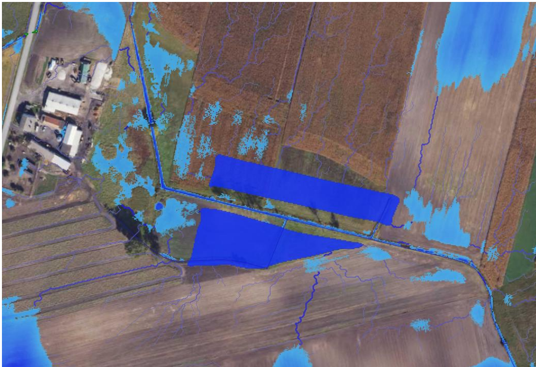
Ryc. 6.4.1.5. Zasięg zalewu wód w otoczeniu analizowanego cieku w sytuacji funkcjonowania dwóch zbiorników retencyjnych podczas opadów 20 mm
