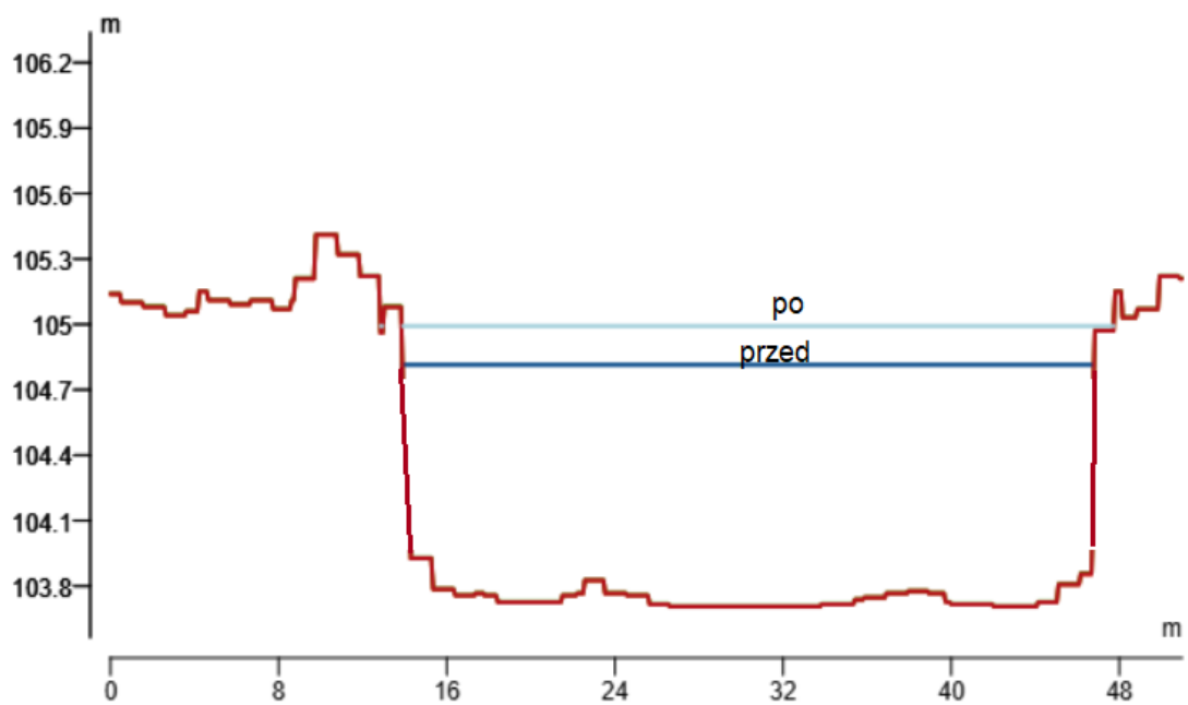
Ryc. 6.4.1.8. Profil podłużny przez czasę zbiornika wraz z rzędną lustra wody przed i po skierowaniu wód z sąsiedniej zlewni.
