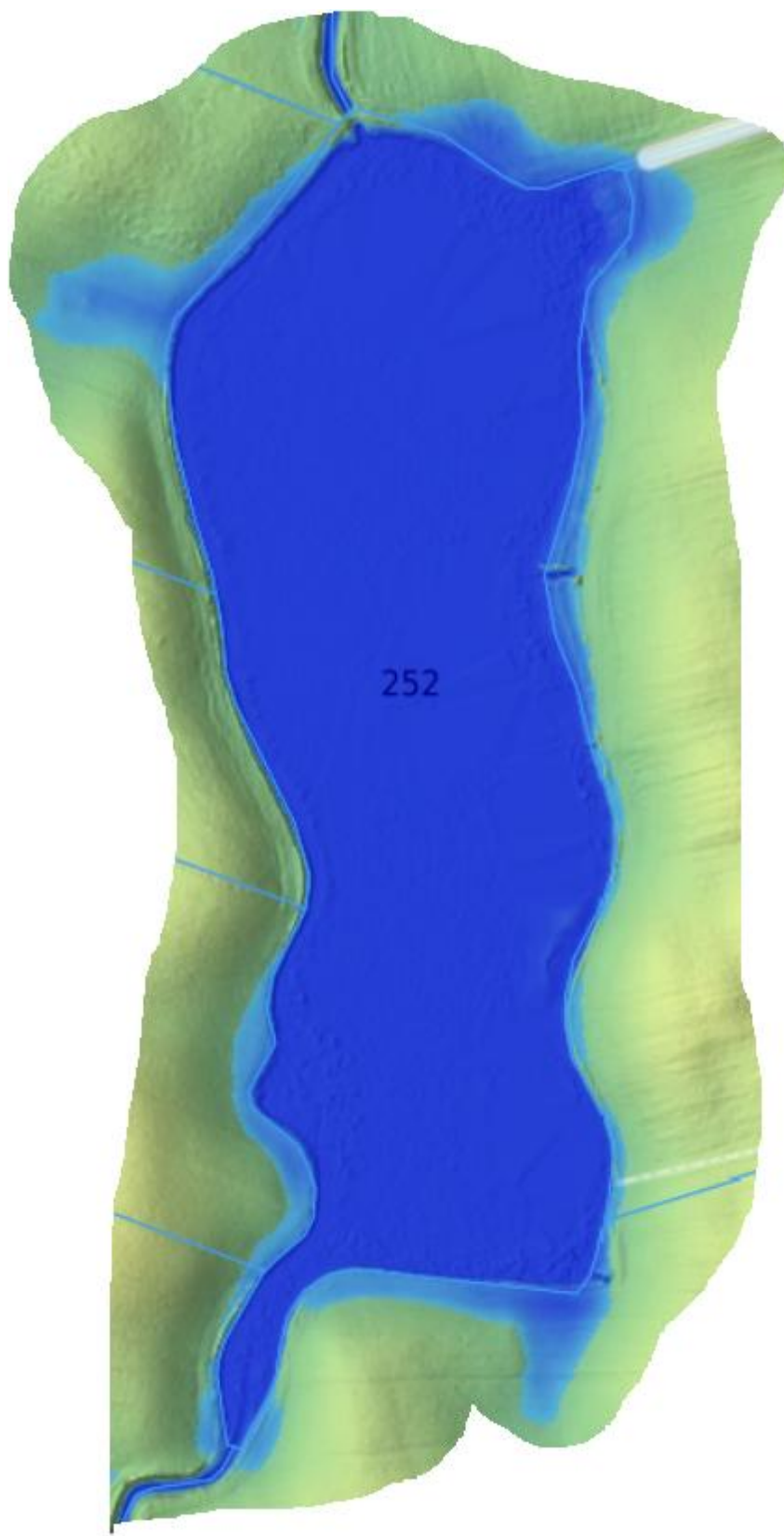
Ryc. 6.4.2.6. Zasięg linii brzegowej jeziora przy ustanowieniu NPP na rzędnej 102,2 m.
