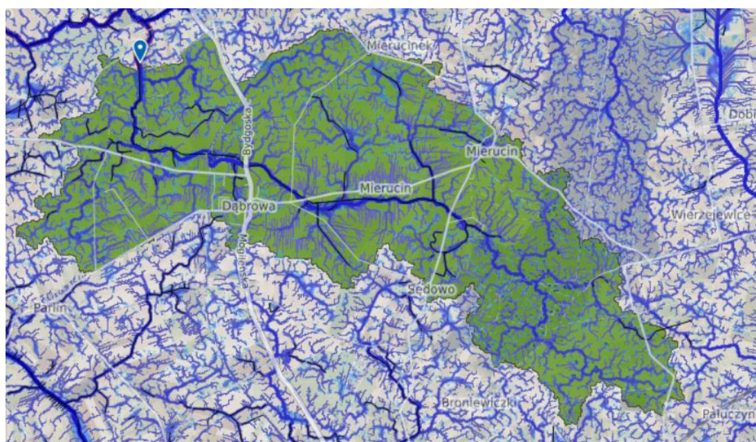
Ryc. 6.4.2.2. Zlewnia Kanału melioracyjnego R-A do profilu wylotu wód z Jeziora Białego.
