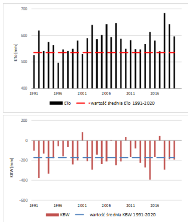
Rys. 2.2.3. Przebieg ETo (mm) i KBW (mm) w Poznaniu i Bydgoszczy w wieloleciu 1991-2020; źródło: ITP-PIB Oddział w Bydgoszczy na podstawie danych IMGW-PIB.
