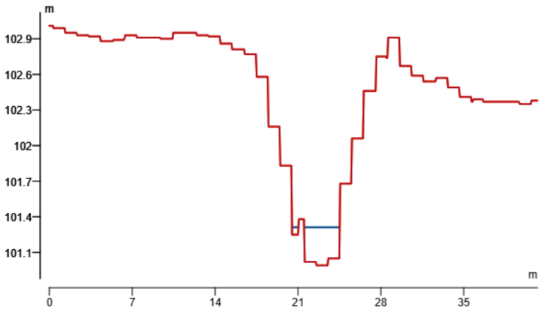
Ryc. 6.4.2.4. Profil poprzeczny na wypływie z jeziora. Dno zastawki jest na rzędnej 100,22. Istnieje możliwość spiętrzenia wód o 2 ma i ustanowienia normalnego poziomu piętrzenia (NPP) na rzędnej 102,20 m
