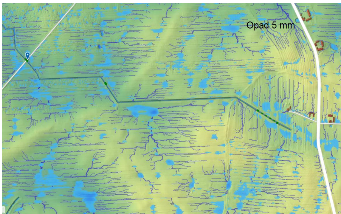
Ryc. 6.4.1.5. Przebieg fragmentu rowu BA1 na tle mapy wysokościowej wraz z siecią drenażu i miejscami kumulacji wód. Rów ma spadek podłużny 1,1 promila (m/km).
