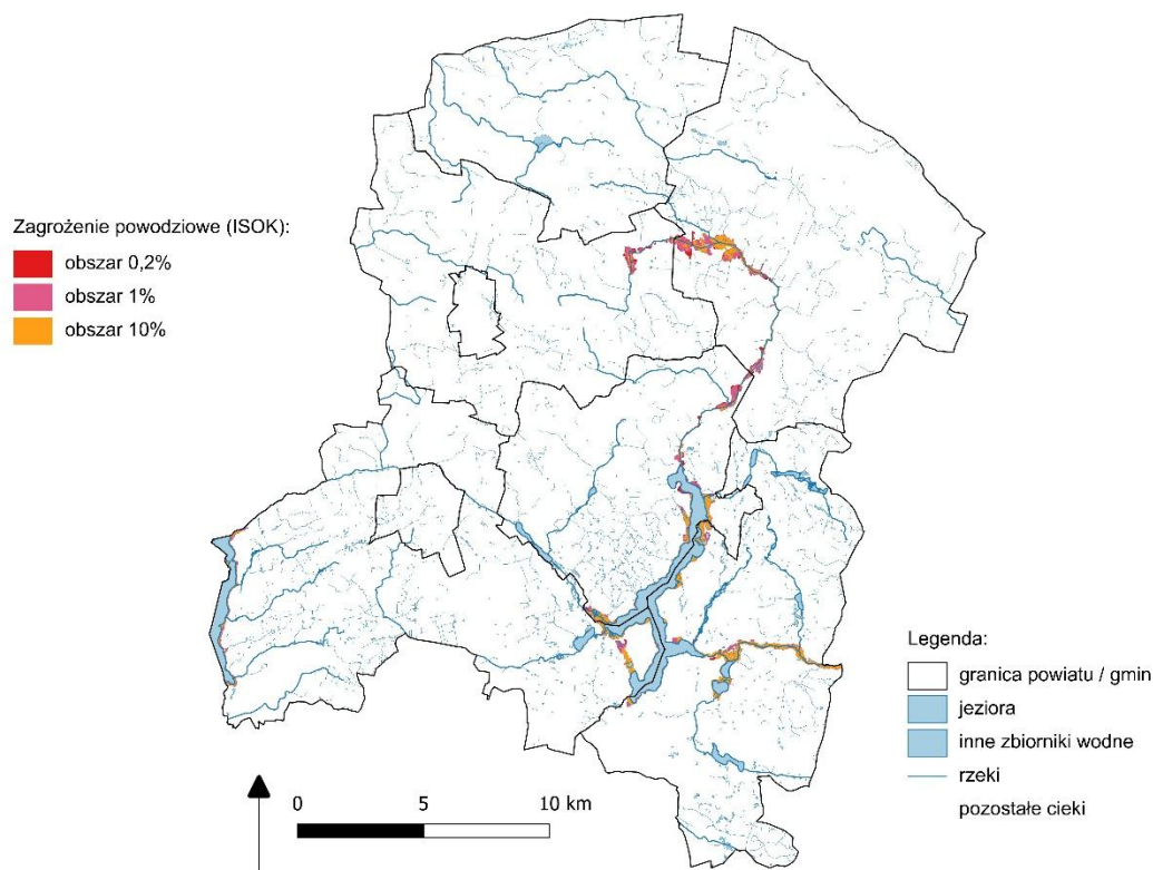
Ryc. 3.3.6. Mapa obszaru zagrożenia powodziowego 0,2%, 1% oraz 10% dla powiatu radziejowskiego, zgodnie z ISOK.
