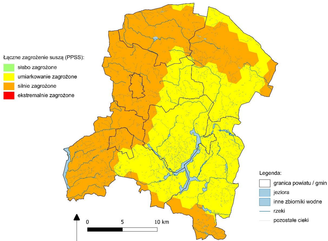
Ryc. 3.3.5. Ocena łącznego zagrożenia suszą na obszarze powiatu radziejowskiego, zgodnie z PPSS.
