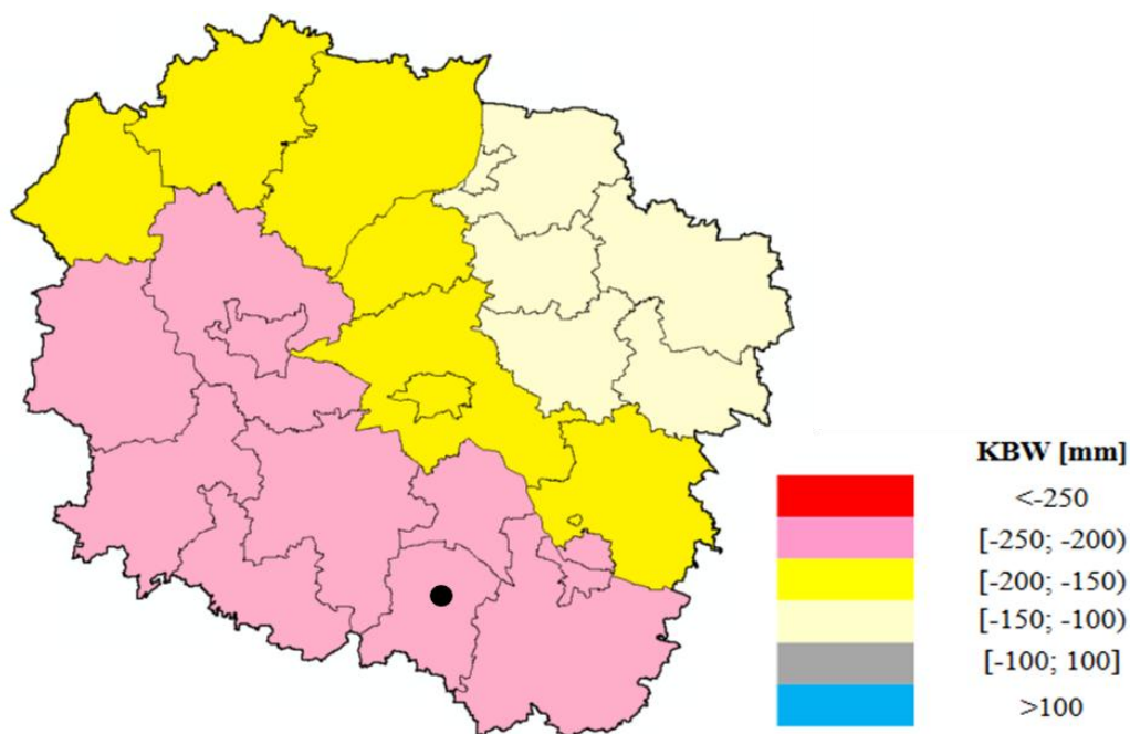
Ryc. 4.2.1. Przestrzenny rozkład klimatycznego bilansu wodnego KBW w okresie wegetacyjnym (kwiecień–wrzesień) w powiecie radziejewskim na tle powiatów woj. kujawsko-pomorskiego; źródło: opracowanie własne na podstawie Łabędzki, 2014
