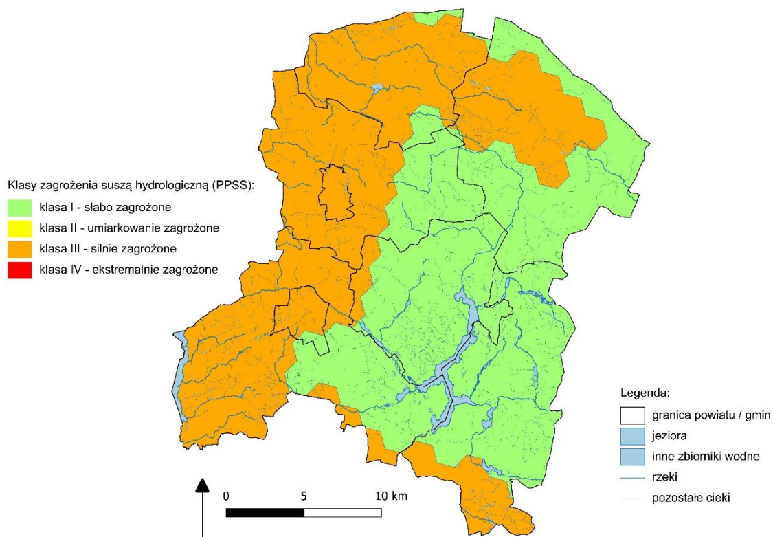
Ryc. 3.3.3. Mapa zagrożenia suszą hydrologiczną na obszarze powiatu radziejewskiego, zgodnie z PPSS.
