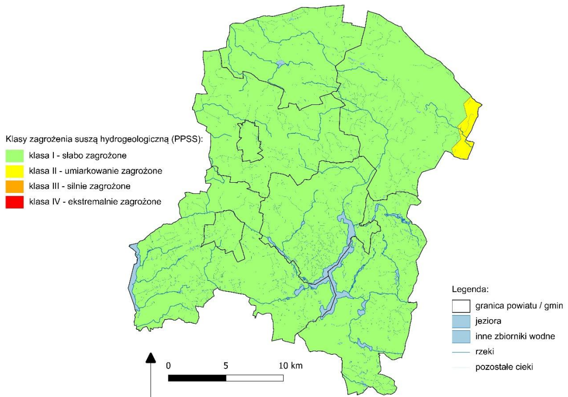
Ryc. 3.3.4. Mapa zagrożenia suszą hydrogeologiczną na obszarze powiatu radziejowskiego, zgodnie z PPSS.
