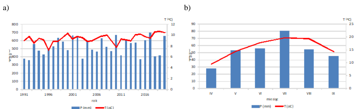
Rys. 1. Przebieg sum opadów atmosferycznych i średniej temperatury powietrza w Bydgoszczy w wieloleciu 1991-2020: a) – w przebiegu rocznym; b) – w okresie wegetacyjnym w wieloleciu 1991-2020. Źródło: ITP Oddział Bydgoszcz
