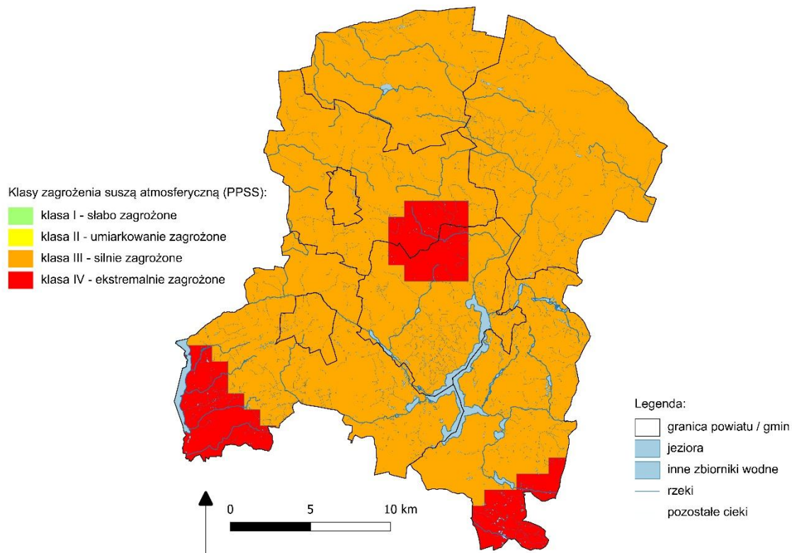
Ryc. 3.3.1. Mapa zagrożenia suszą atmosferyczną na obszarze powiatu radziejewskiego, zgodnie z PPSS.
