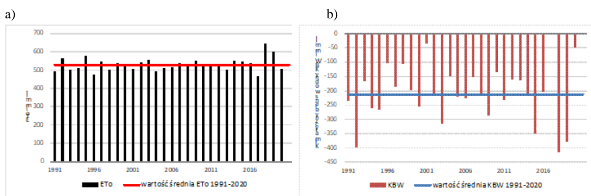
Rys. 3. Charakterystyki sezonu wegetacyjnego (IV-X) w Bydgoszczy w wieloleciu 1991-2020: a) - sumy ewapotranspiracji wskaźnikowej ETo (mm); b) – wartości klimatycznego bilansu wodnego (KBW) (mm). Źródło: ITP Oddział Bydgoszcz
