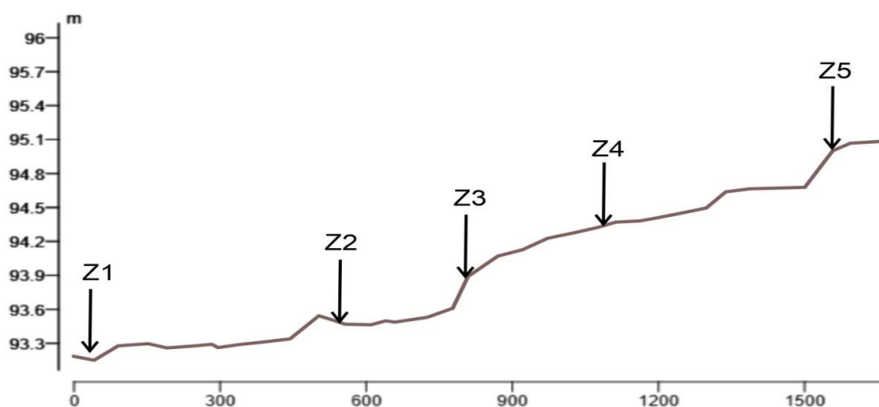
Ryc. 6.4.1.6. Profil podłużny hipsometryczny terenu wzdłuż analizowanego odcinka rowu BA1.
