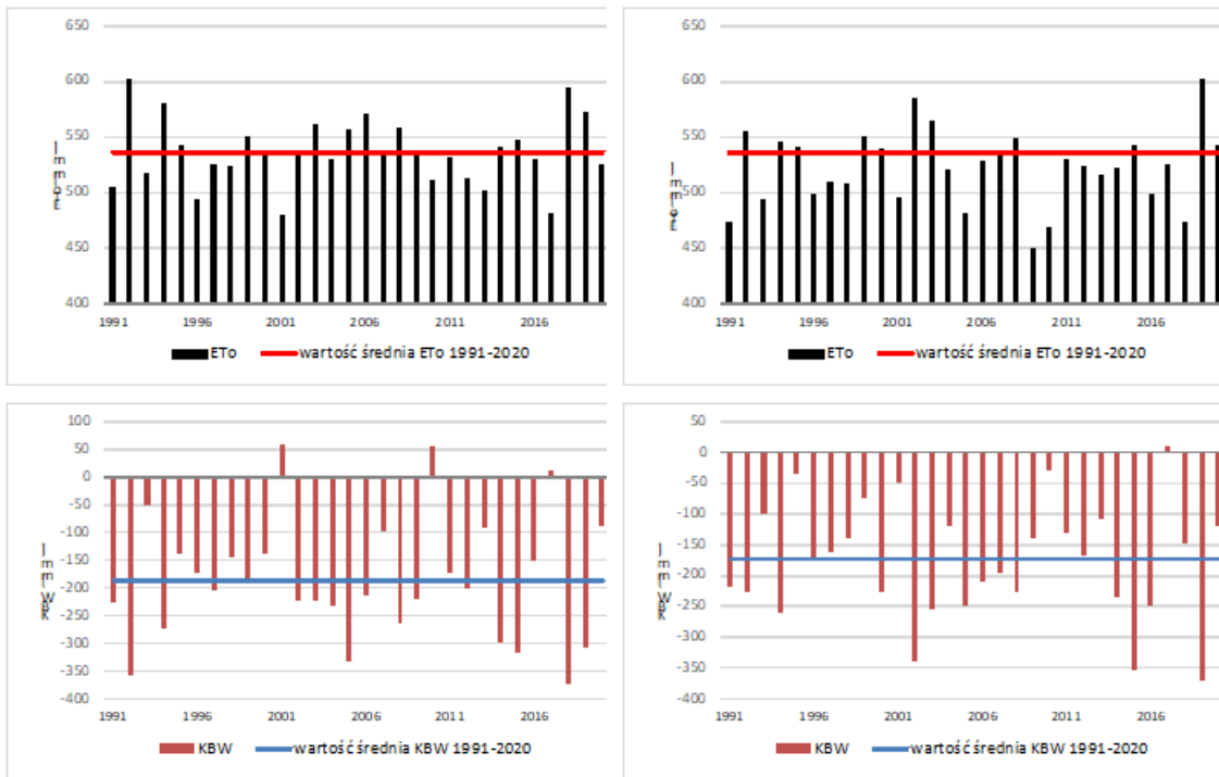
Rys. 2.2.4. Przebieg ETo i KBW (mm) w Toruniu i Mławie w wieloleciu 1991-2020. źródło: ITP-PIB Oddział w Bydgoszczy na podstawie danych IMGW-PIB
