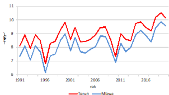
Rys. 2.2.3. Przebieg temperatury w Toruniu i Mławie w wieloleciu 1991-2020: a) średnia roczna temperatura, b) średnia temperatura w okresie wegetacyjnym (IV-IX). źródło: ITP-PIB Oddział w Bydgoszczy na podstawie danych IMGW-PIB
