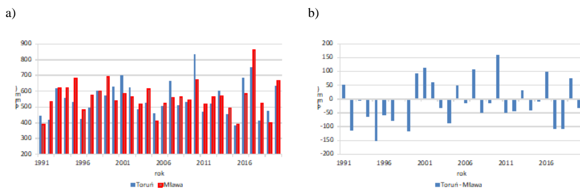
Rys. 2.2.1. Przebieg opadów w Toruniu i Mławie w wieloleciu 1991-2020: a) roczne sumy opadów atmosferycznych, b) różnice rocznych sum; źródło: ITP-PIB Oddział w Bydgoszczy na podstawie danych IMGW-PIB
