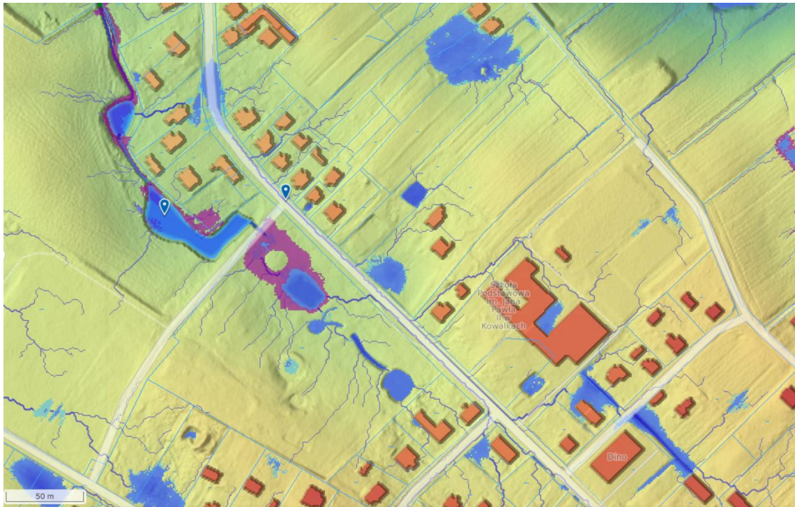
Ryc. 6.4.1.6. Mapa prezentująca porównanie warunków splywu wód powierzchniowych i zasięgu podtopień przed (fioletowy kolor) i po budowie zbiorników: Park, proj. Zbiornik 1 i Zbiornik 2 – ścieżki i kierunki splywu przy opadzie 40 mm w obrębie projektowanej inwestycji.
