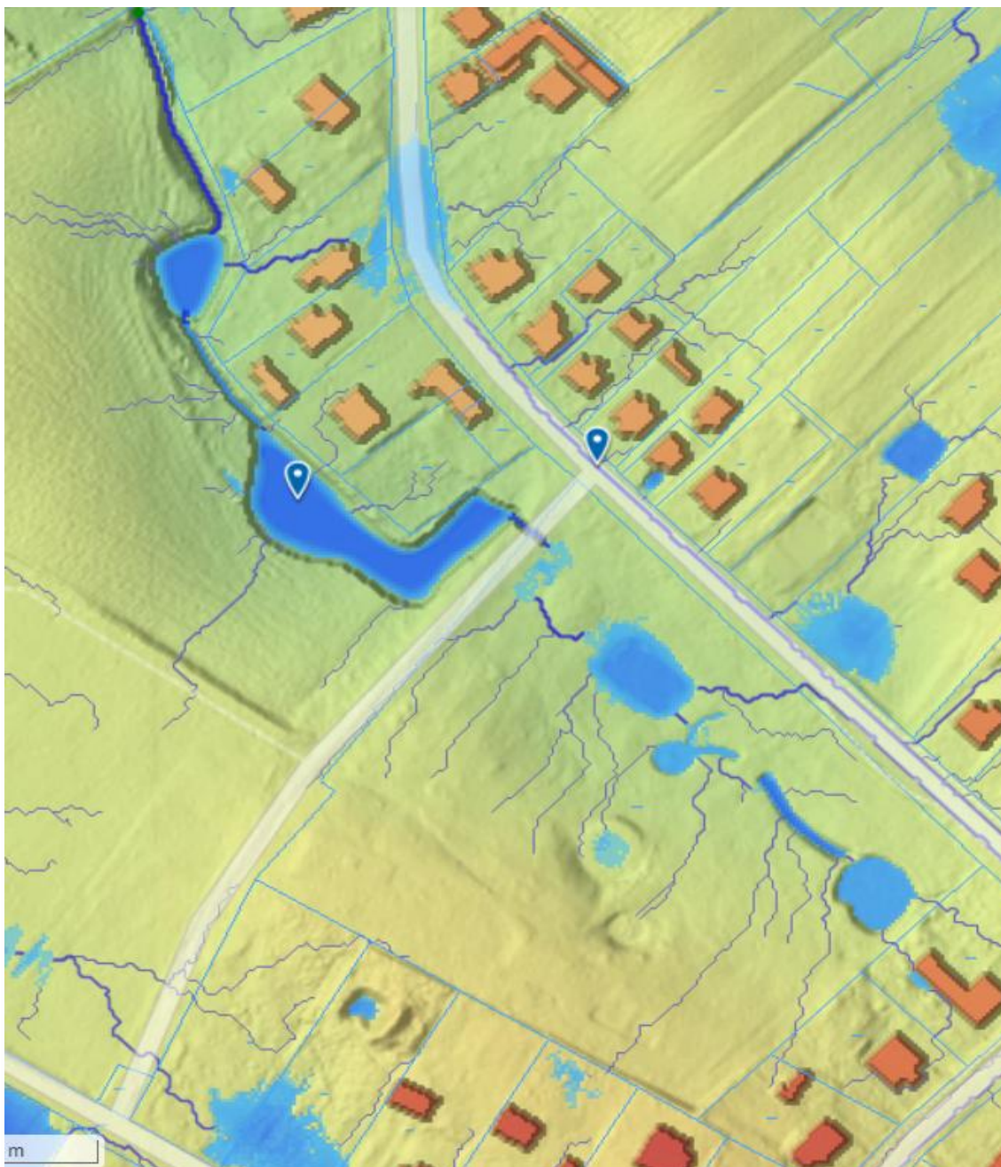
Ryc. 6.4.1.5. Mapa prezentująca warunki spływu wód powierzchniowych: Park, proj. Zbiornik 1 i Zbiornik 2 – ścieżki i kierunki spływu przy opadzie 40 mm w obrębie projektowanej inwestycji.
