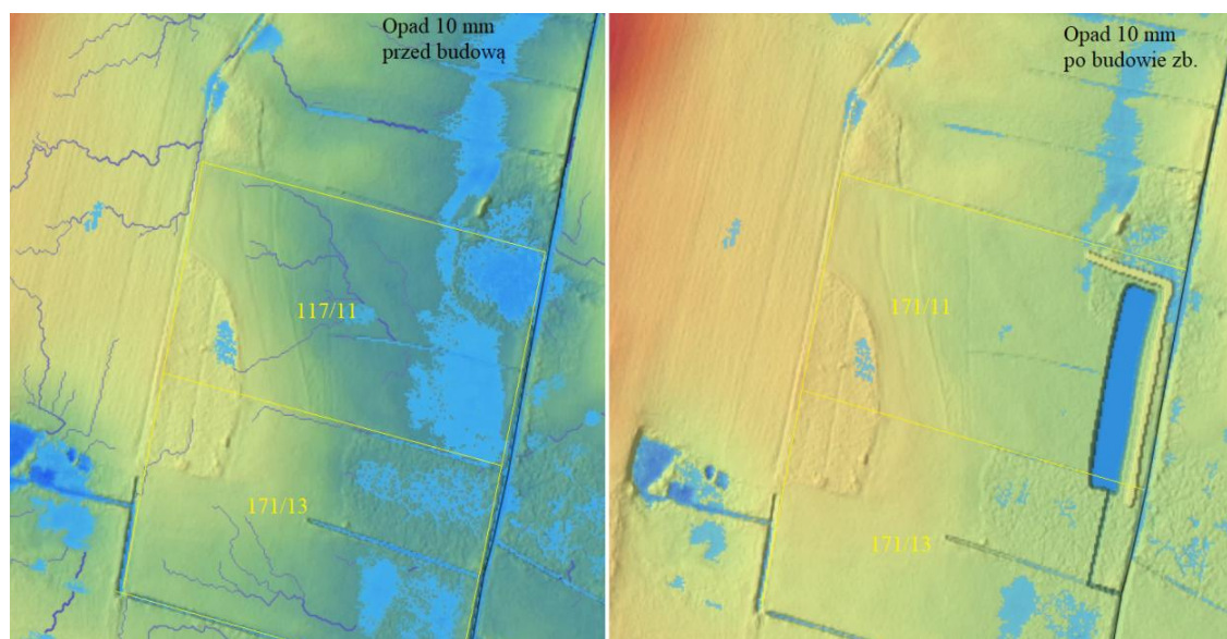
Ryc. 6.4.1.9. Wariant 2. Budowa zbiornika wraz z groblą (rzędna korony 96,3 m) oddzielającą działkę 171/1 od wód Strugi Granicznej, 50 m odcinek rowu na połączeniu ze Strugą.
